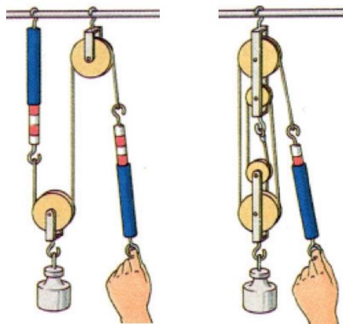
Abb. 9: Flaschenzug
